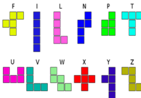
Рис. 3 Пентамино
