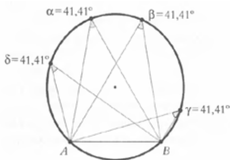
Рис. 1. Окружность
