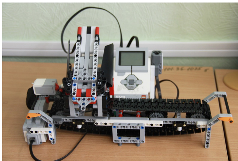
Рис. 3. Робот-сортировщик
