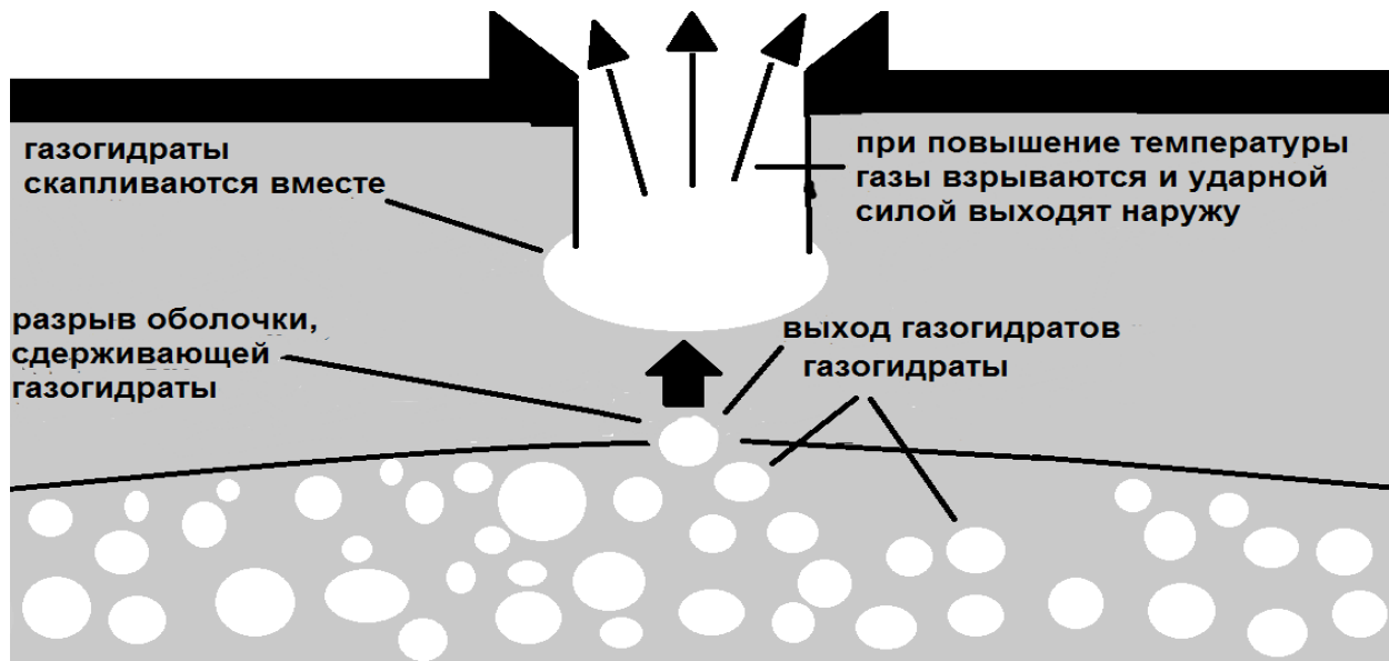
Рис. 4. Схема выброса газогидратов на поверхность Земли
