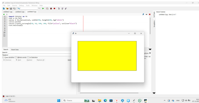
Рис. 1. Создание прямоугольника в Python
