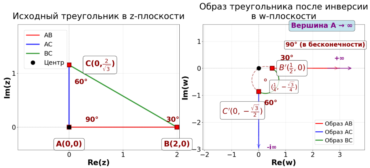
Рис. 8. Преобразования треугольника при инверсии (создан с Python)
