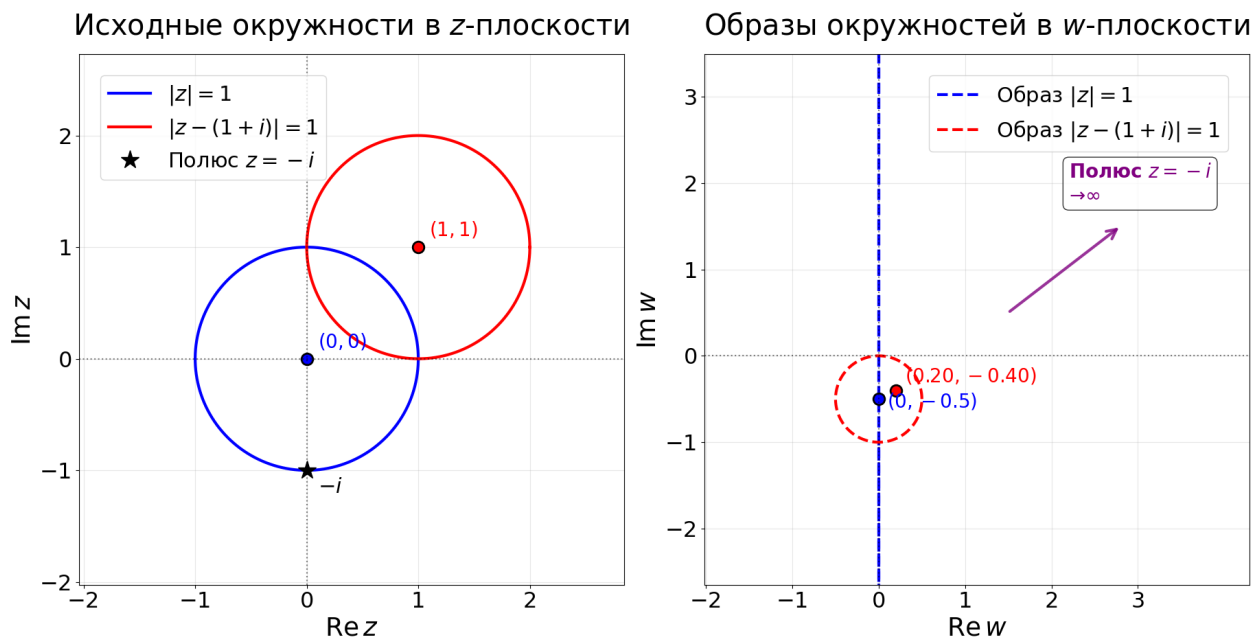
Рис. 11. Преобразование окружностей (создан с Python)
