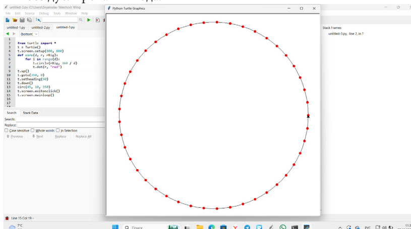
Рис. 6. Круг с заданным количеством точек
