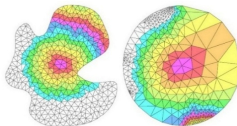
Рис.2. Визуализация теоремы Римана о отображении
