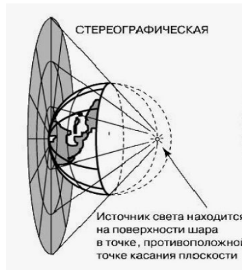
Рис. 1. Пример стереографической проекции (рисунок взят из Сети)
