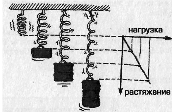
Рис. 2. Связь между растяжением пружин и действующими на них нагрузками
