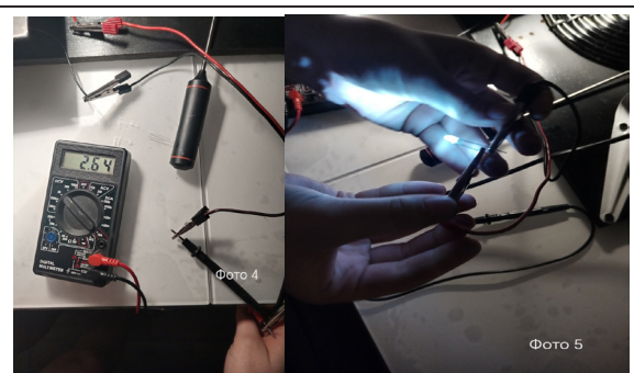
Рис. 5. Финальный эксперимент
