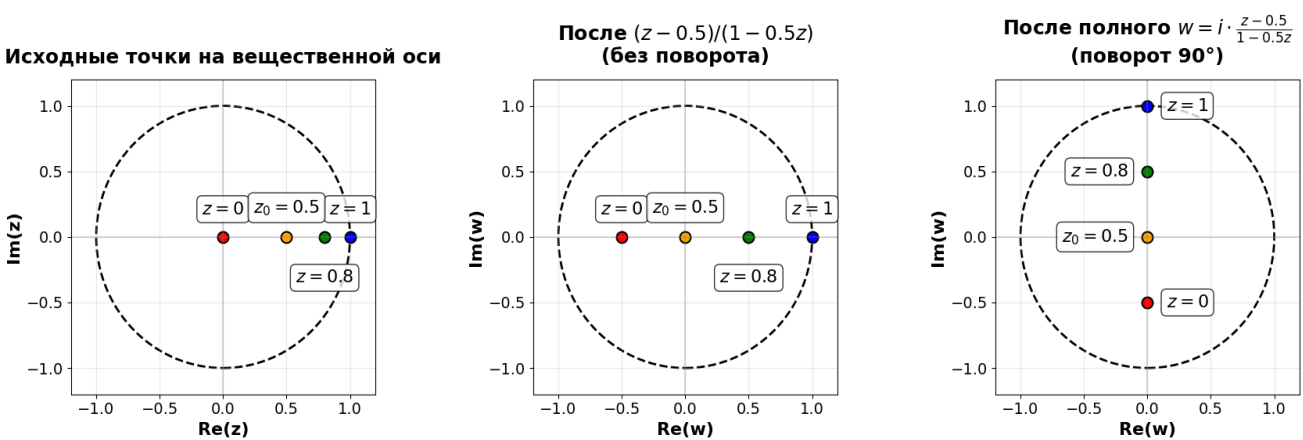
Рис. 15. Отражение единичного круга на единичный круг (создан с Python)
