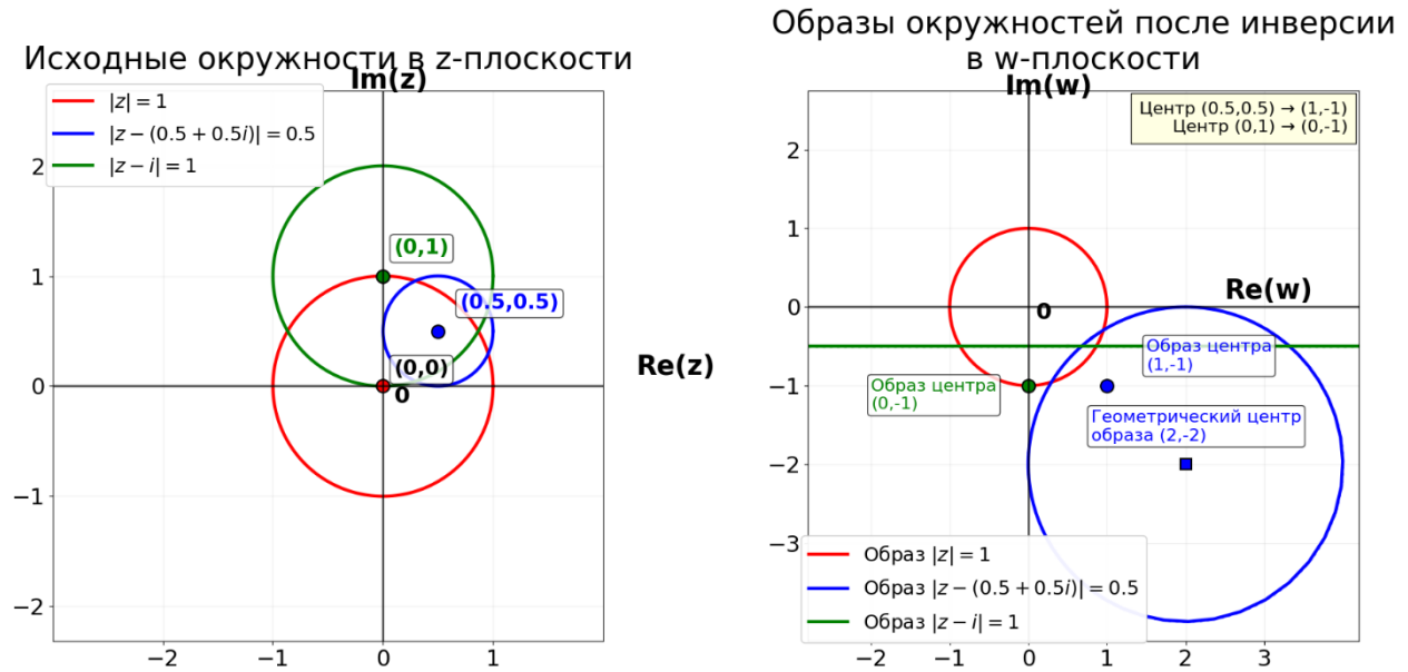
Рис. 7. Преобразования окружностей при инверсии (создан с Python)
