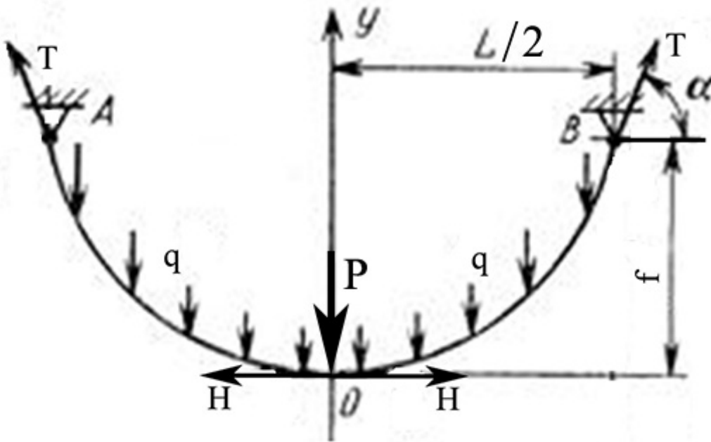
Рис. 1. Расчетная схема
