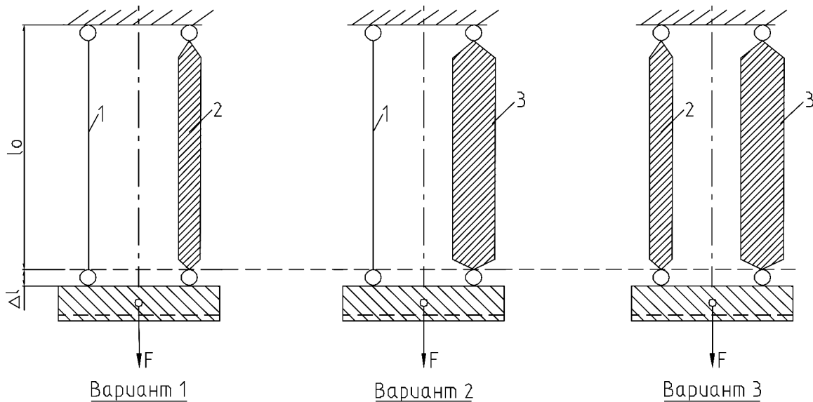
Рис. 3. Схема нагружения параллельных стержней из различных материалов при их одинаковом удлинении (первоначальная длина l_0 = 1 м, сила F = 20 кН)
