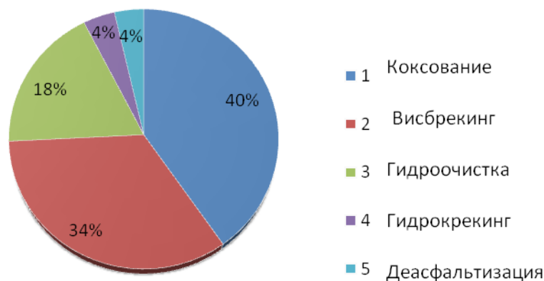
Рис. 1. Доля различных процессов в мировой переработке тяжёлой нефти
