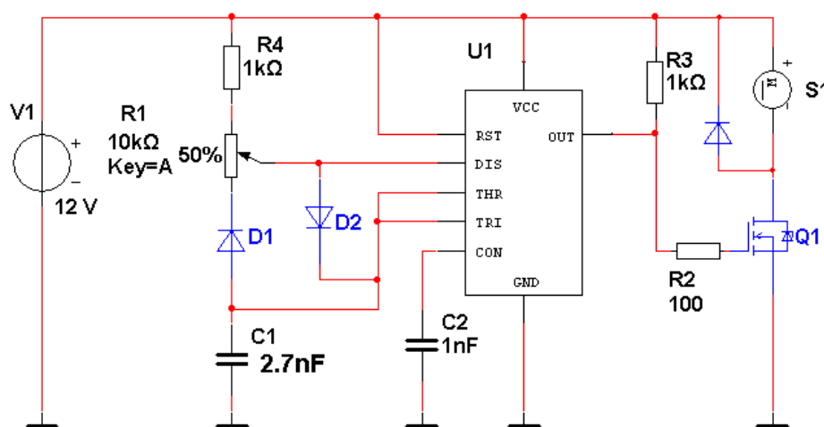
Рис. 2. Схема стандартного широтно-импульсного регулятора оборотов
