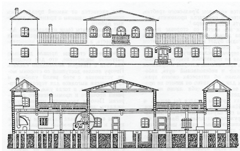
Рис. 3. Чертеж Завода для выделки сырых, оленьих шкур в замшу (из книги Летопись Севера (1964 г.))
